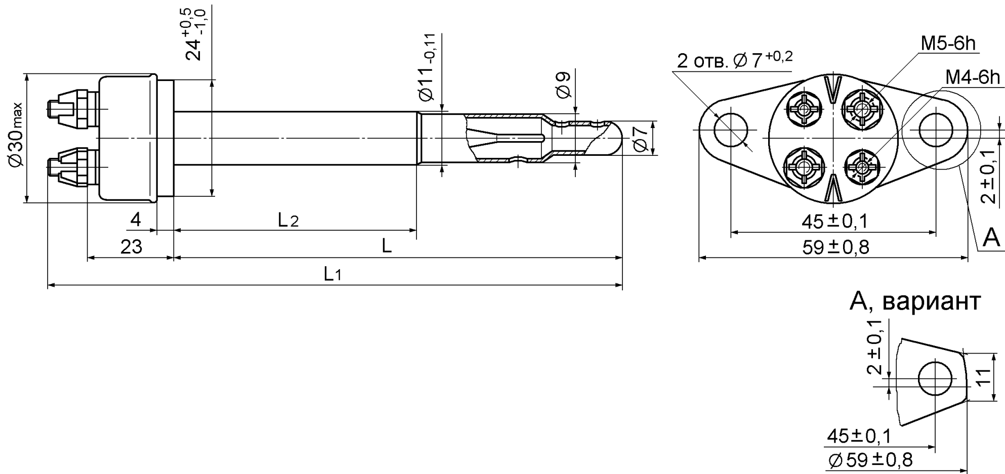
Рисунок 2 – Габаритный чертеж термопреобразователей ТХА-75К, ТХА-100К
