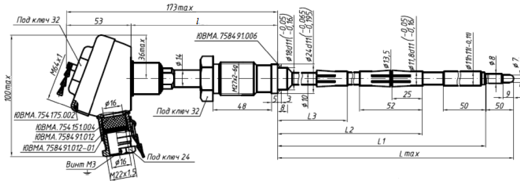
Рисунок В.2 – Штуцер подвижный
