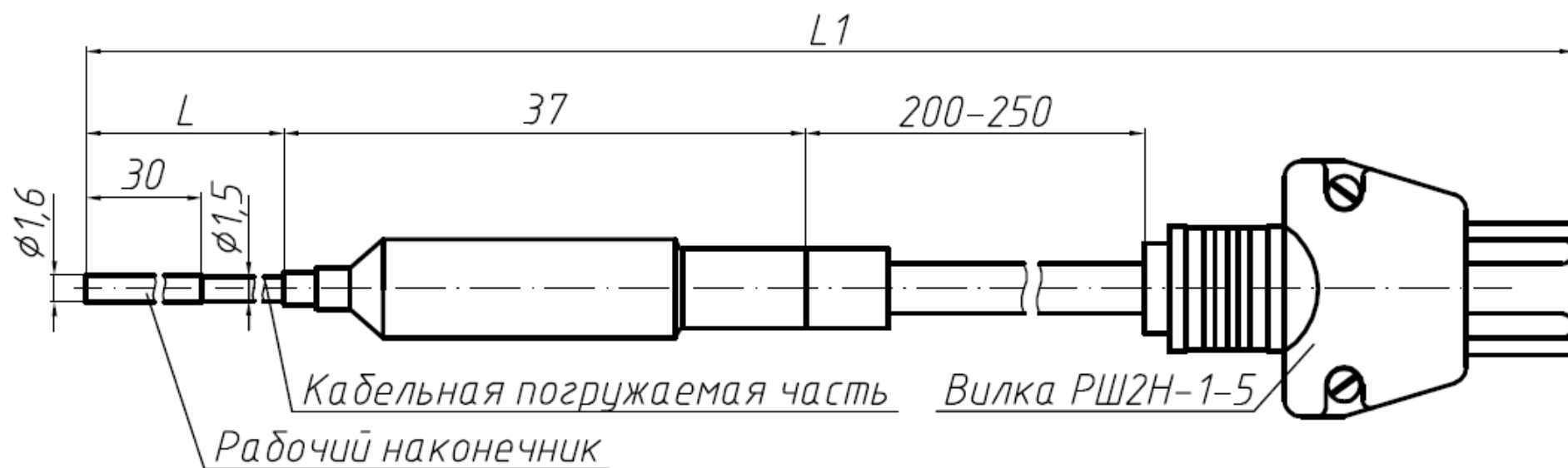
Габаритные чертежи термометров ТСП-ОМ
