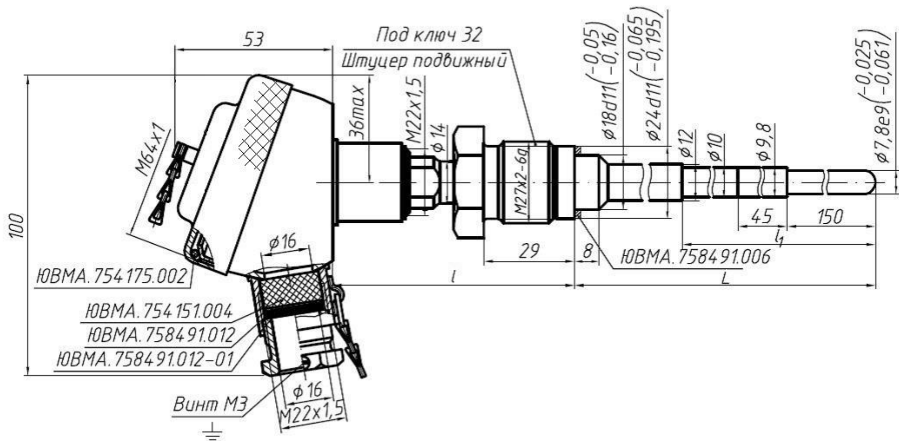
Рисунок Г.2 – Штуцер подвижный
