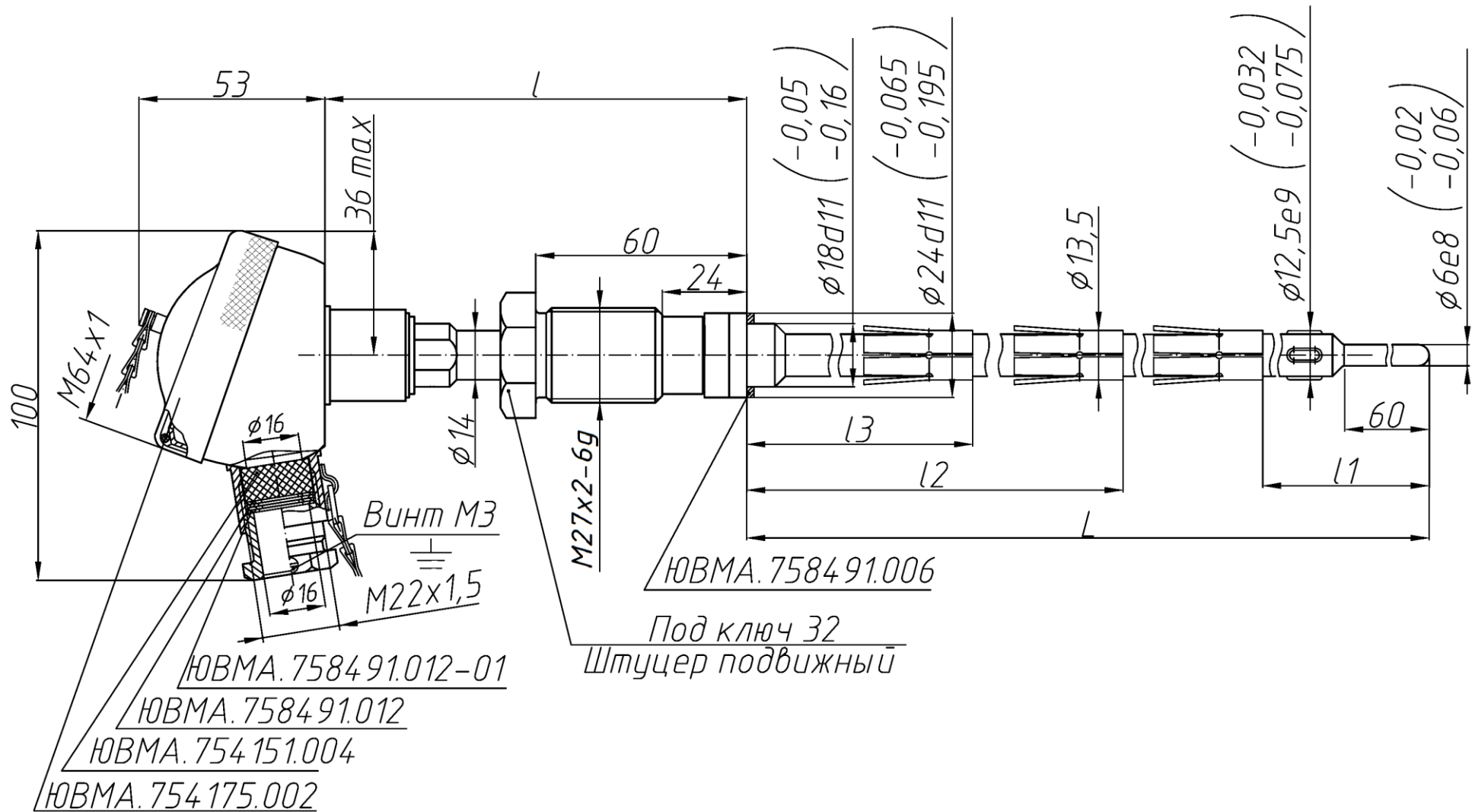
Рисунок Г.1 – Штуцер подвижный
