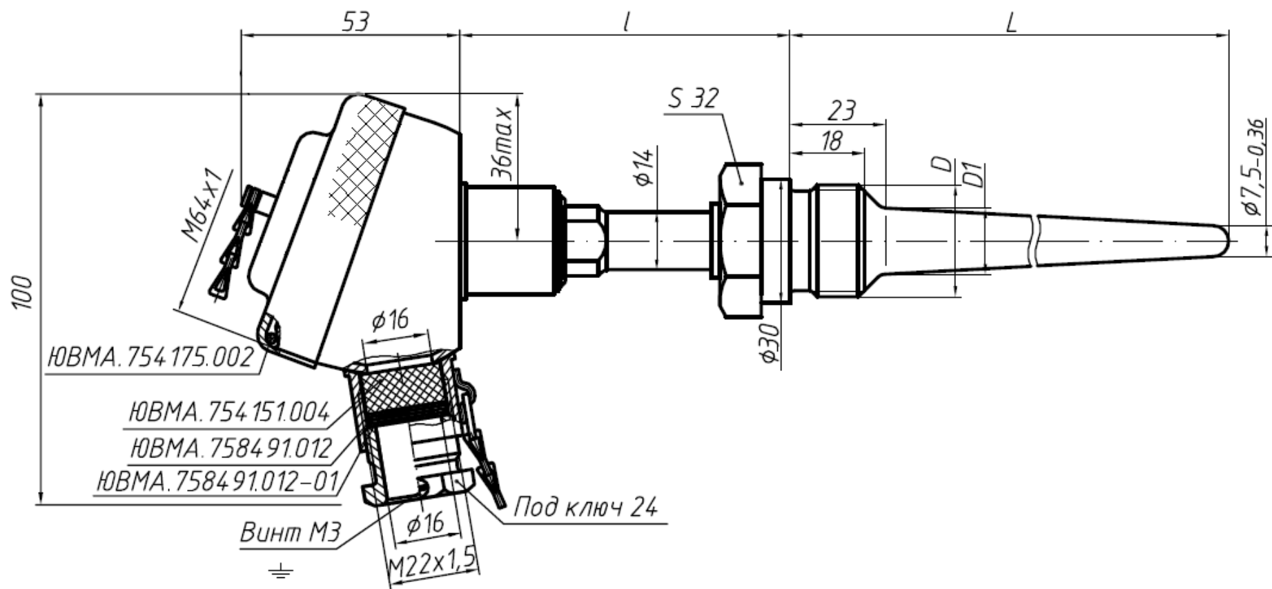
Рисунок В.8 – Штуцер неподвижный
