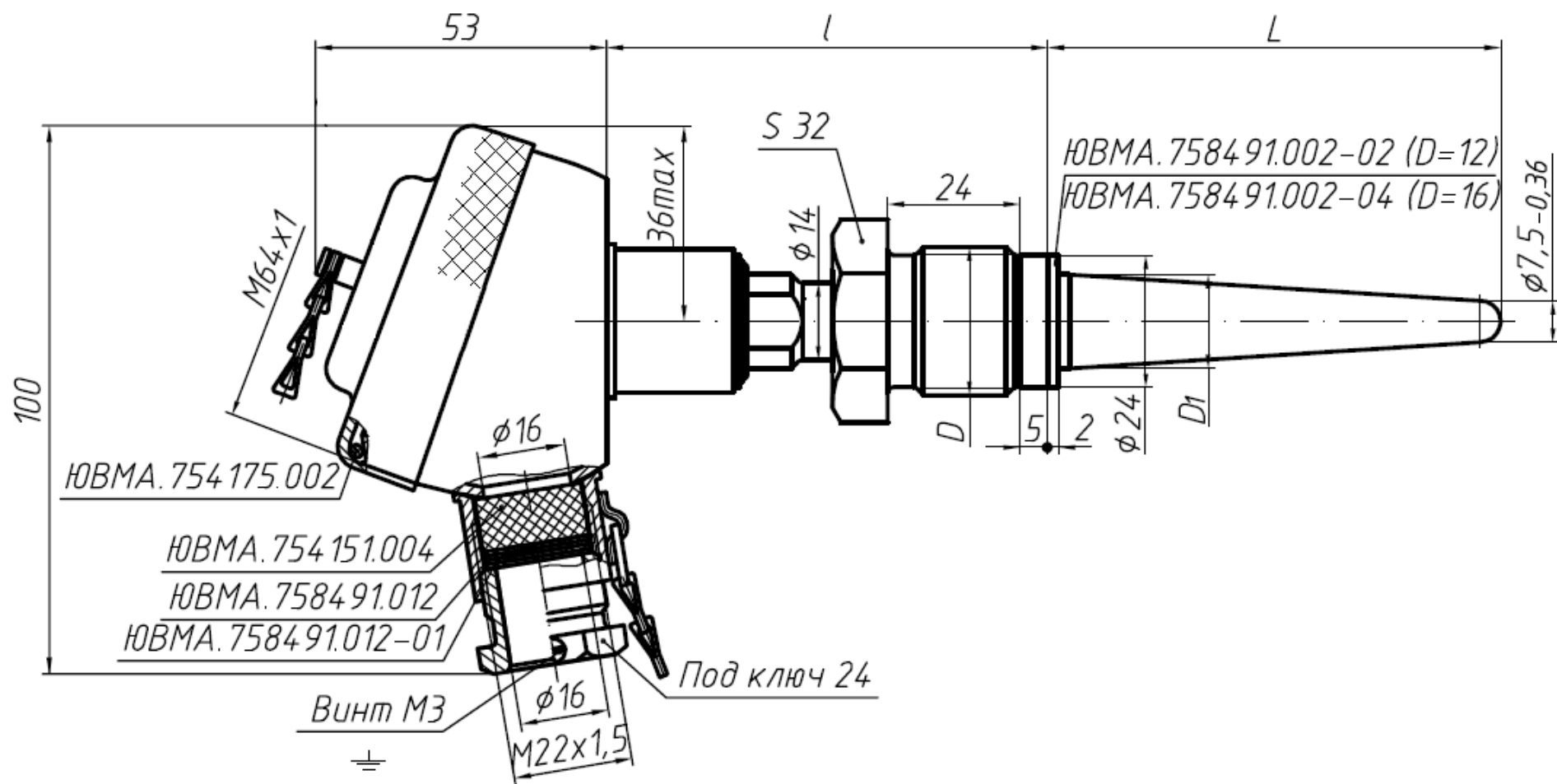
Рисунок В.7 – Штуцер подвижный
