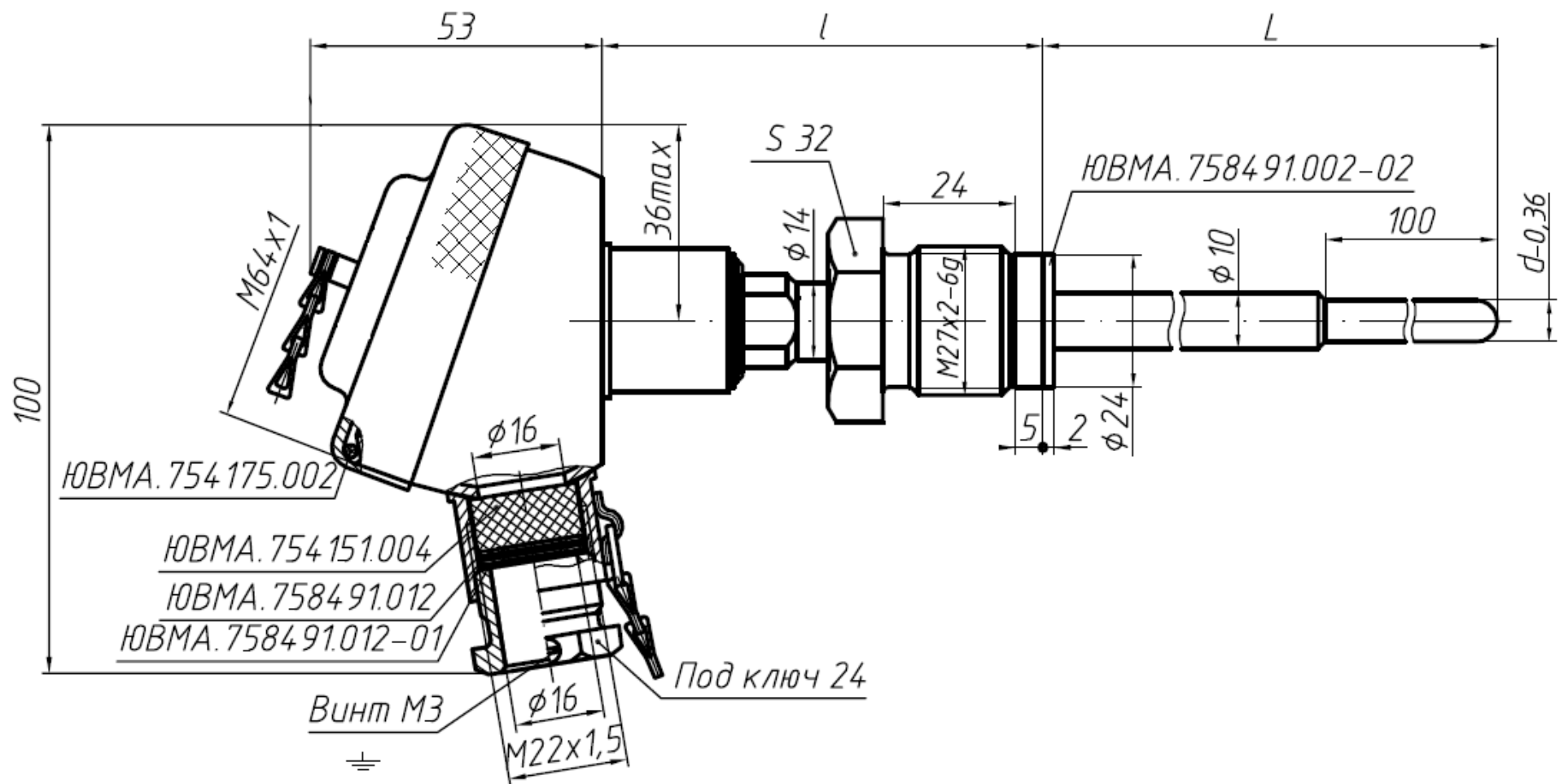
Рисунок В.6 – Штуцер подвижный
