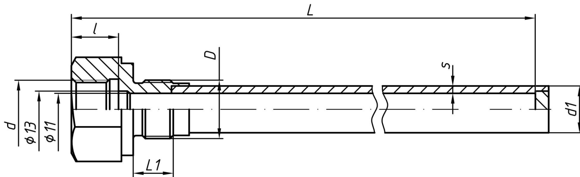
Рисунок 8 – Гильза ГЗШ – 4
