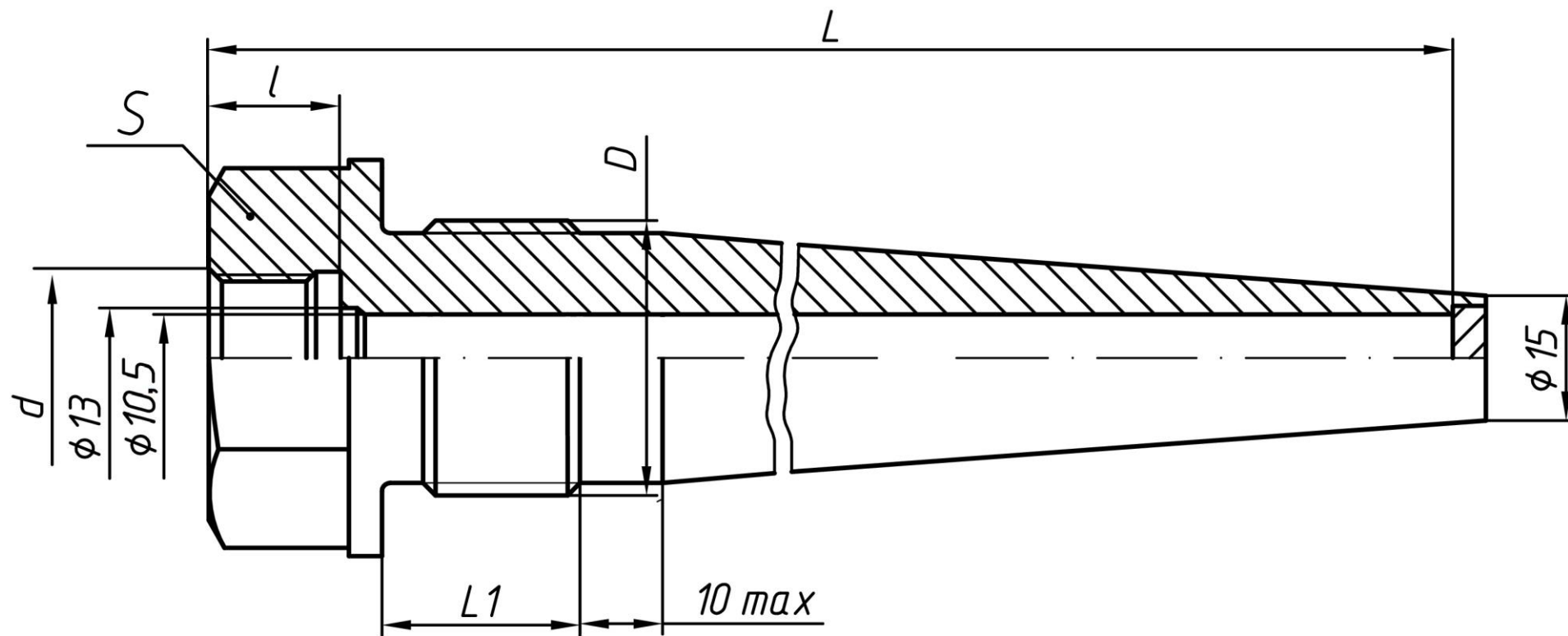
Рисунок 6 – Гильза ГЗШ – 2
