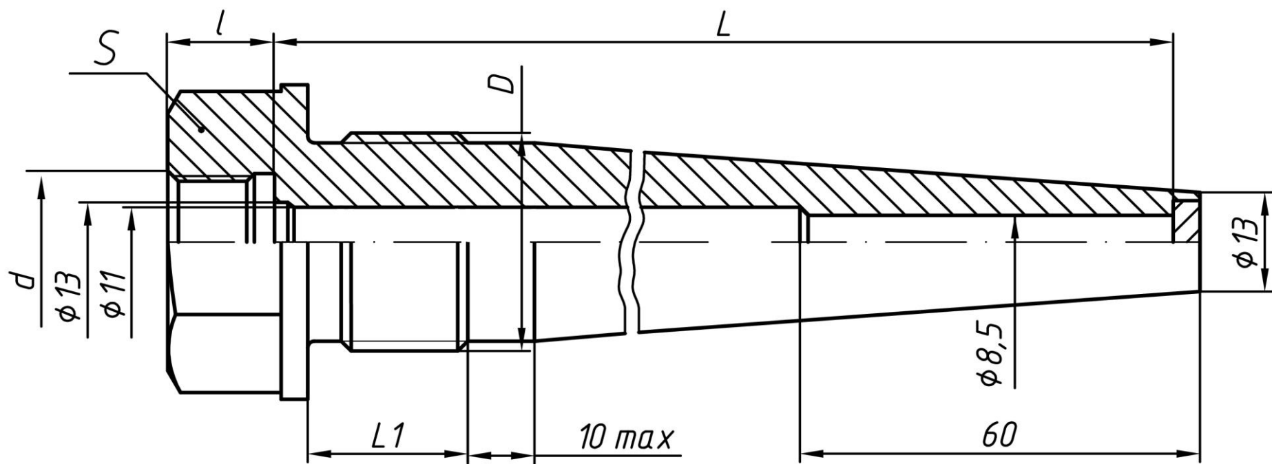
Рисунок 1 - ГЗШ-1
