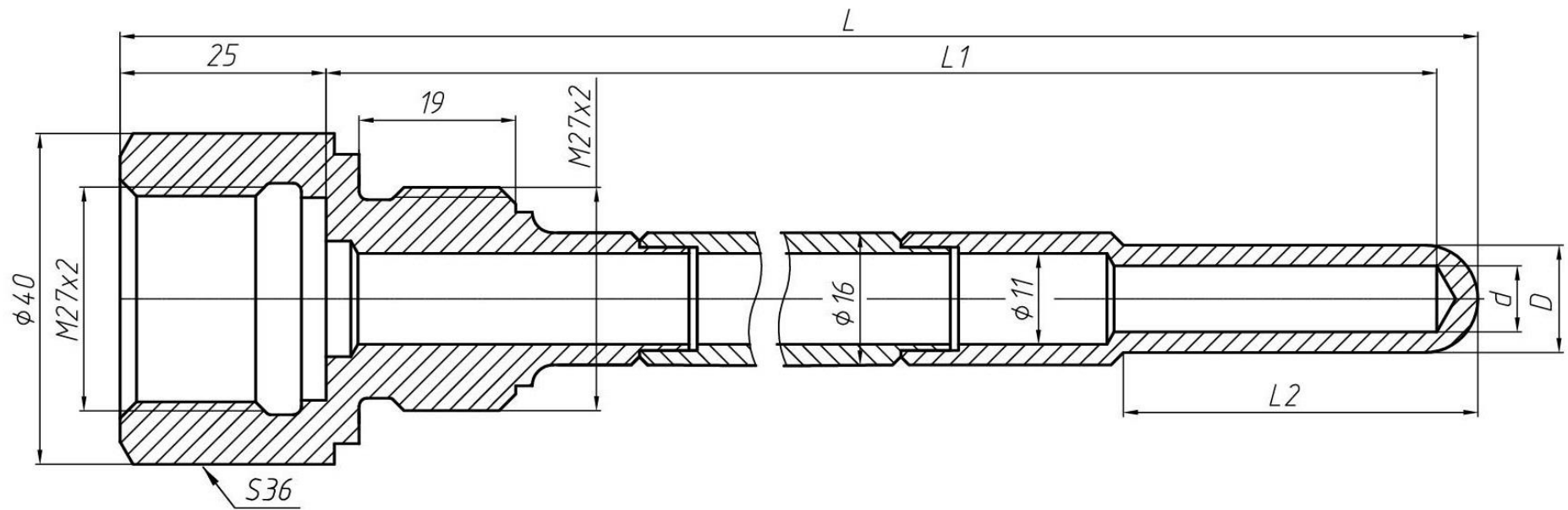
Рисунок 14 – Гильза ГЗШ-8040 (ЮВМА.408721.154) (для датчиков температуры с подвижным и неподвижным штуцером)
