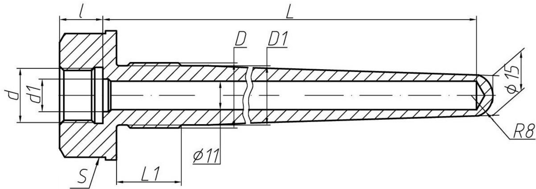
Рисунок 12 - ГЗШ-2Ц, ГЗШ-2Ц Н (ГЗШ-2Ц - ЮВМА.408721.159-072...-101; ГЗШ-2Ц Н - ЮВМА.408721.159-102...-143)
