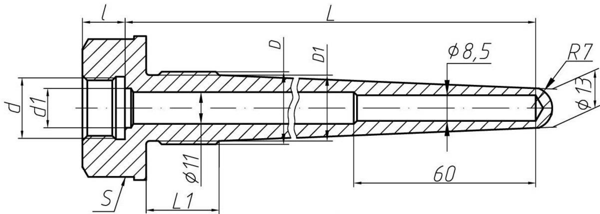
Рисунок 11 - ГЗШ-1Ц, ГЗШ-1Ц Н (ГЗШ-1Ц - ЮВМА.408721.159-000...-029; ГЗШ-1Ц Н - ЮВМА.408721.159-030...-071)
