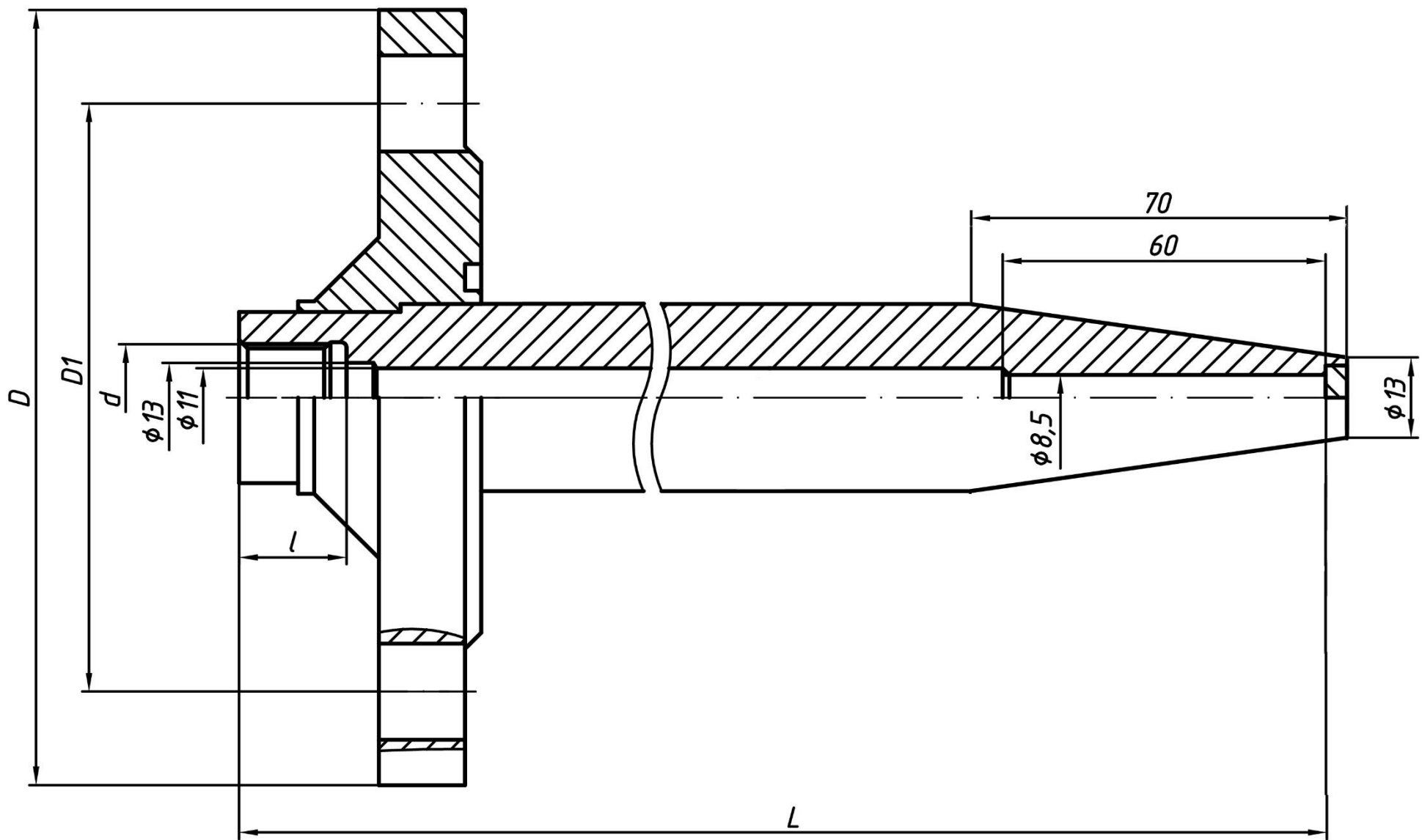
Рисунок 6 – Гильза ГЗФ - 3
