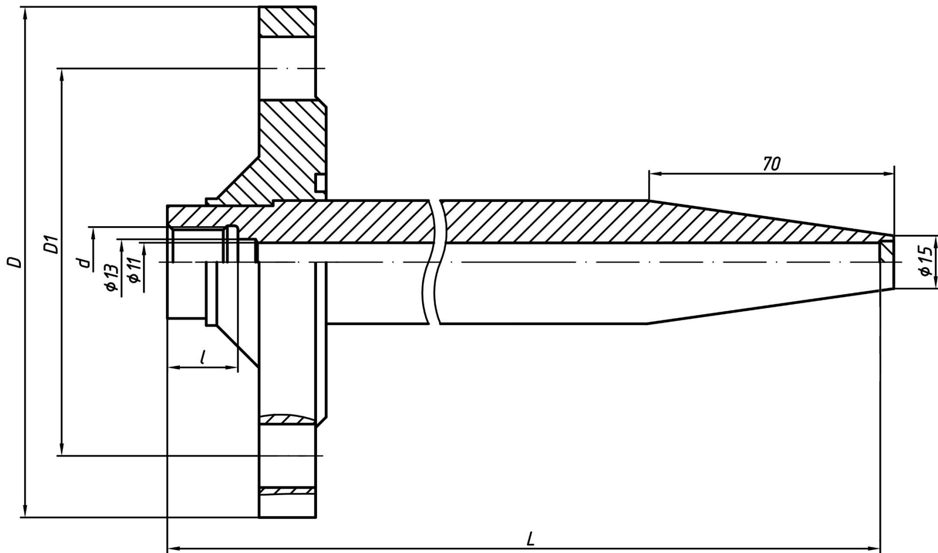
Рисунок 5 – Гильза ГЗФ - 2
