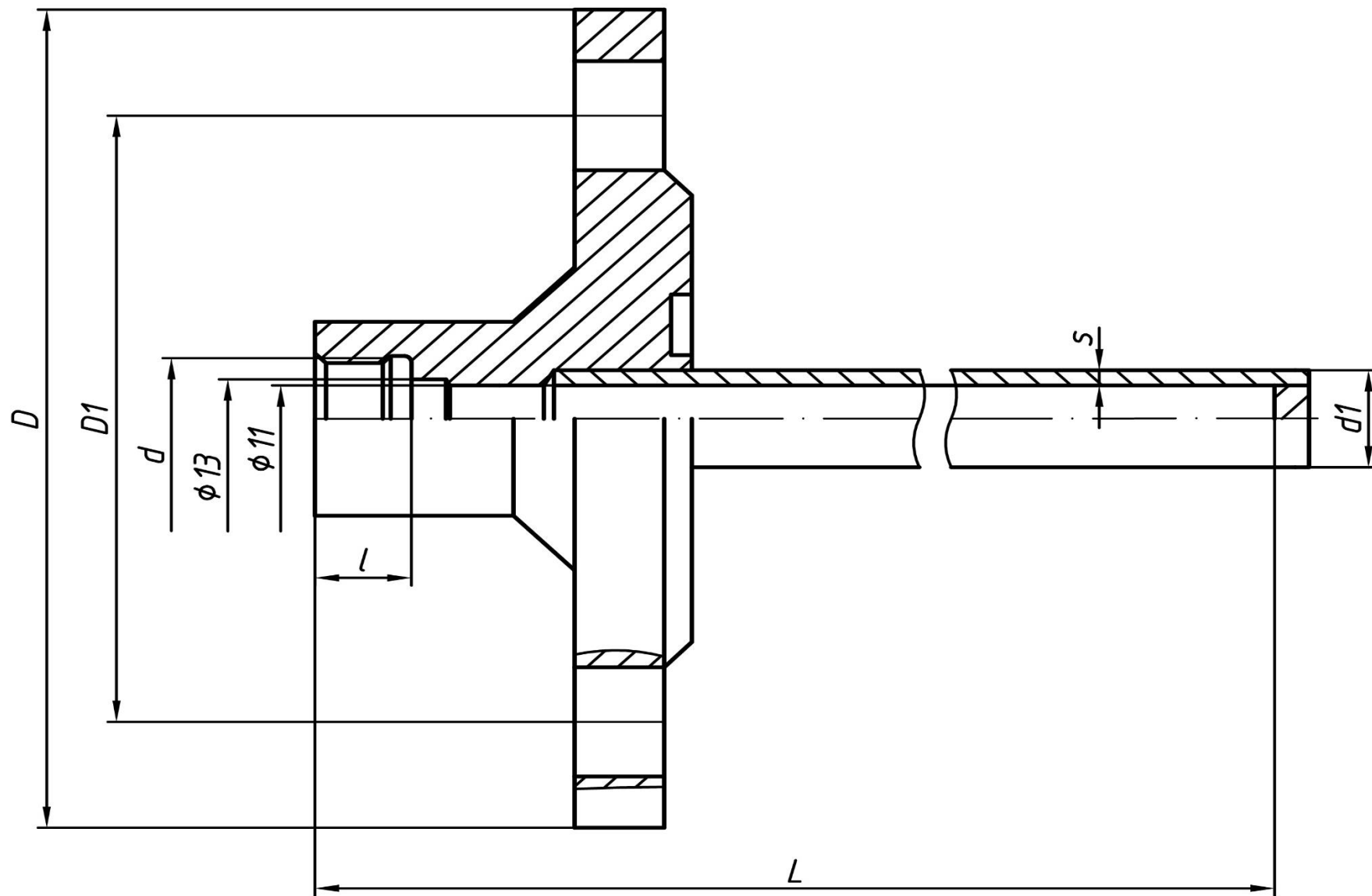
Рисунок 4 – Гильза ГЗФ - 1
