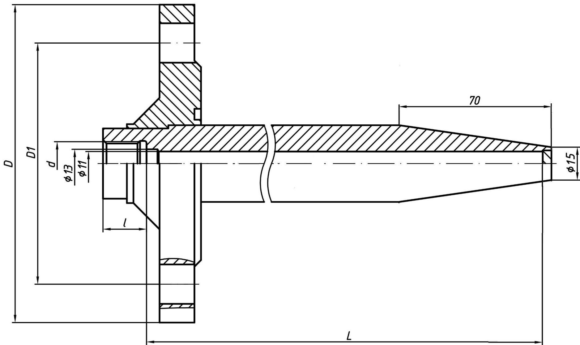
Рисунок 2 – Гильза ГЗФ - 2
