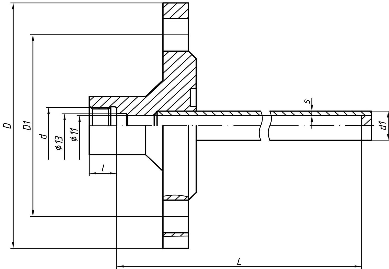
Рисунок 1 – Гильза ГЗФ - 1
