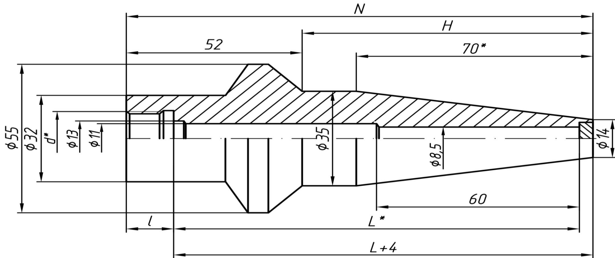
Рисунок 2 – Гильза ГЗВ - 2
