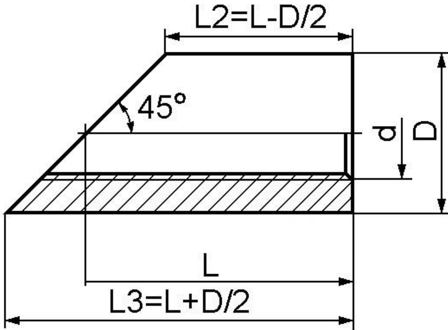
Рисунок 4 – Бобышка тип 4 (под неподвижный штуцер)
