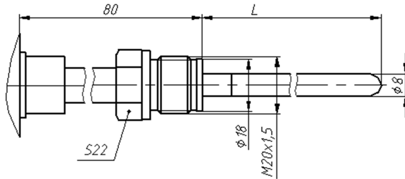
Рисунок Н.3 Штуцер подвижный. Остальное – см. рисунок Н.1
