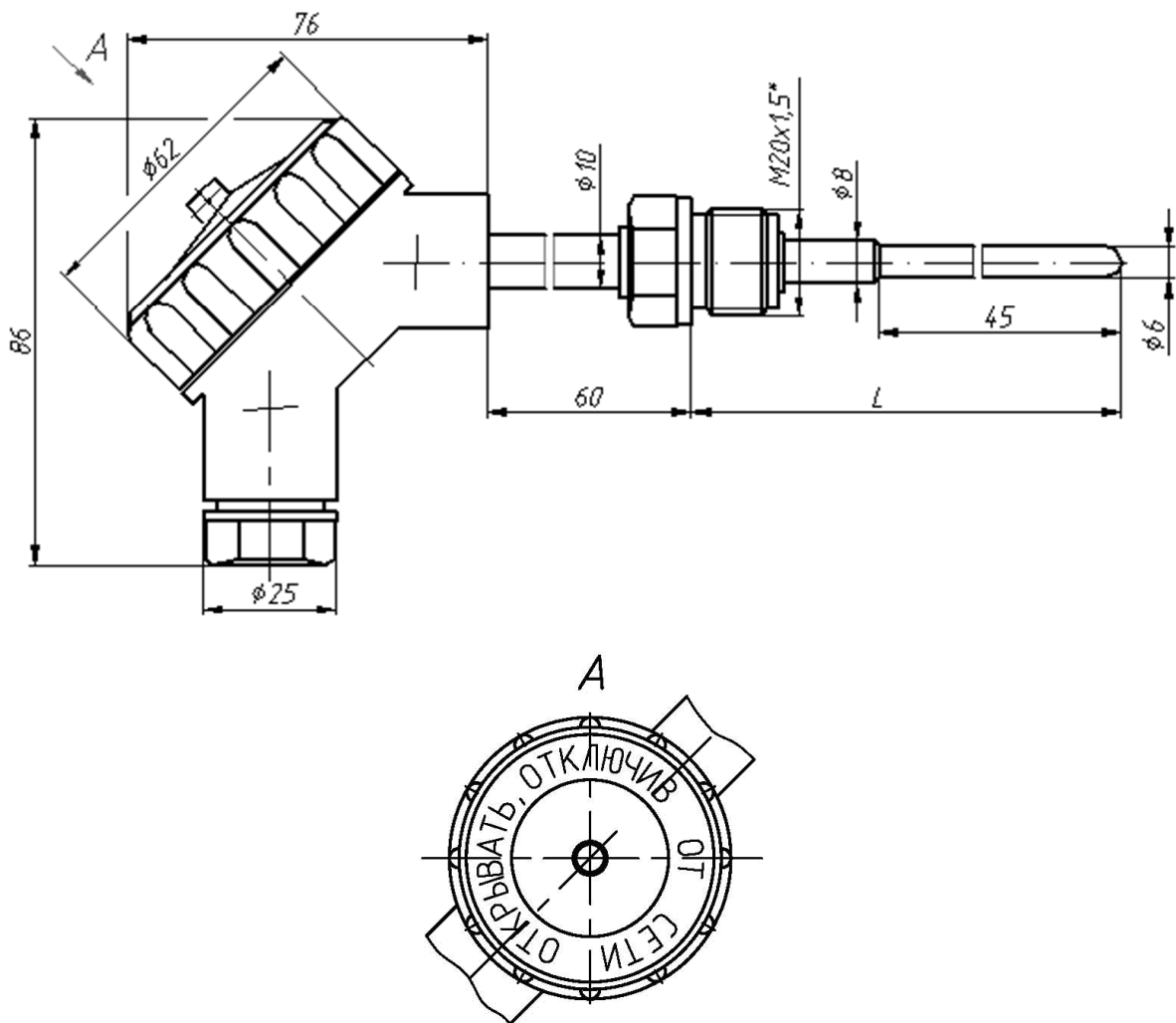
Рисунок Н.11 Штуцер неподвижный, пластмассовая головка (пресс-материал ДСВ-2-0 или АГ-4В). Защитная арматура – с заужением.
