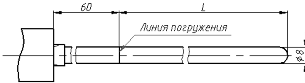
Рисунок Н.14 - Защитная арматура – без заужения, без крепежного штуцера.
