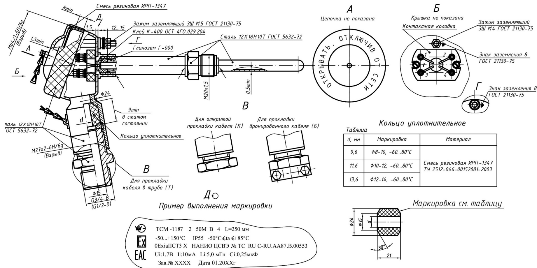
Рисунок А.1 – Чертеж средств взрывозащиты термопреобразователей с головкой из нержавеющей стали и видом взрывозащиты «i»
