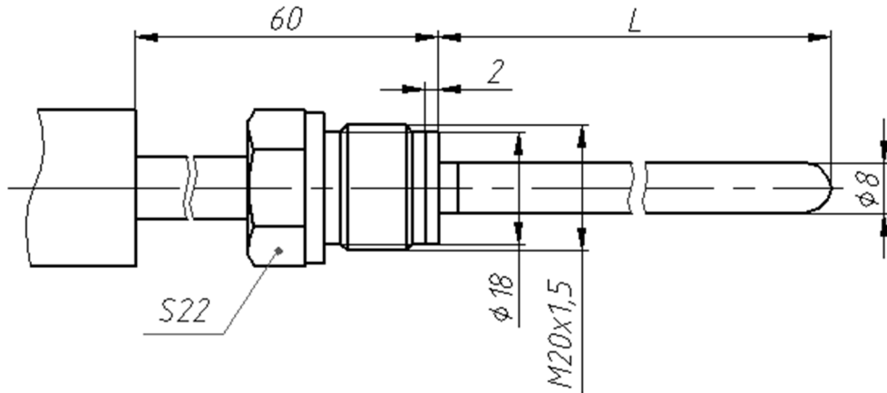
Рисунок Н.13 Защитная арматура – без заужения, штуцер подвижный.
