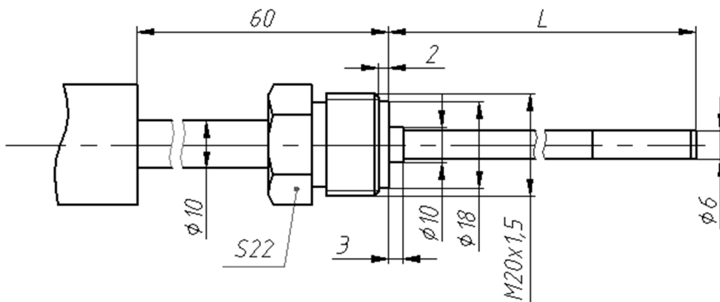
Рисунок Н.15 Защитная арматура – кабельная (вариант 1), штуцер подвижный.
