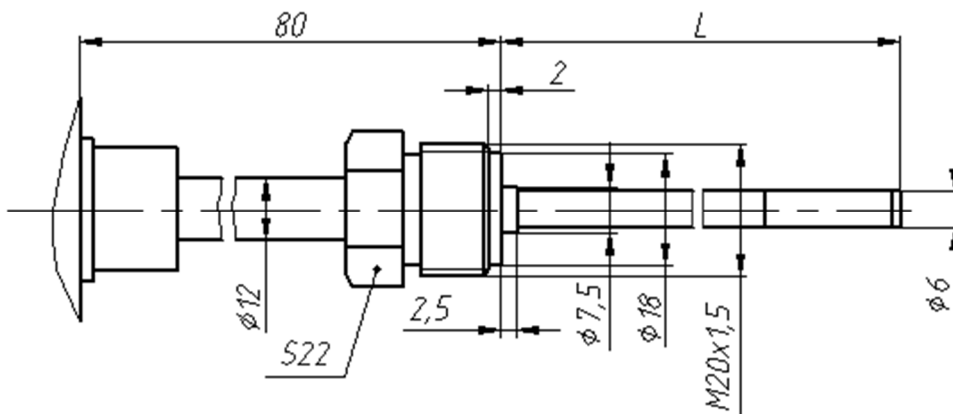
Рисунок Н.5 Штуцер подвижный. Остальное – см. рисунок Н.1
