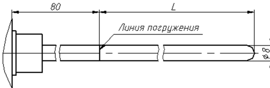
Рисунок Н.4 Без крепежного штуцера. Остальное – см. рисунок Н.1
