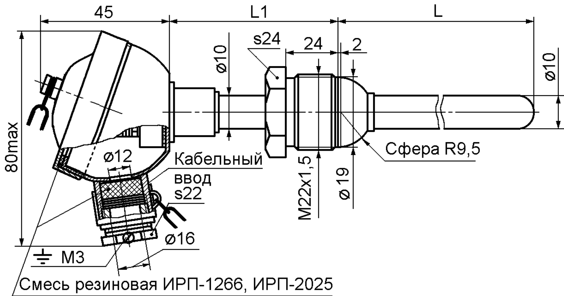
Рисунок Г.9 – Штуцер подвижный
