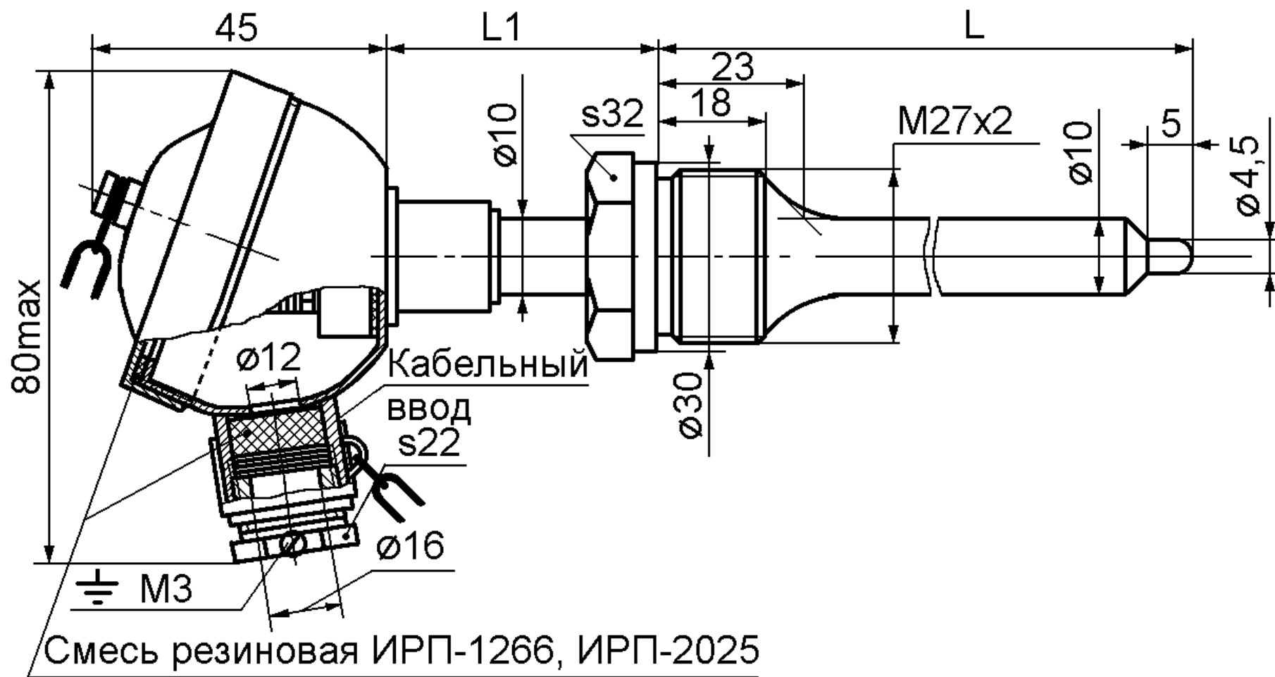
Рисунок Г.7 – Штуцер неподвижный
