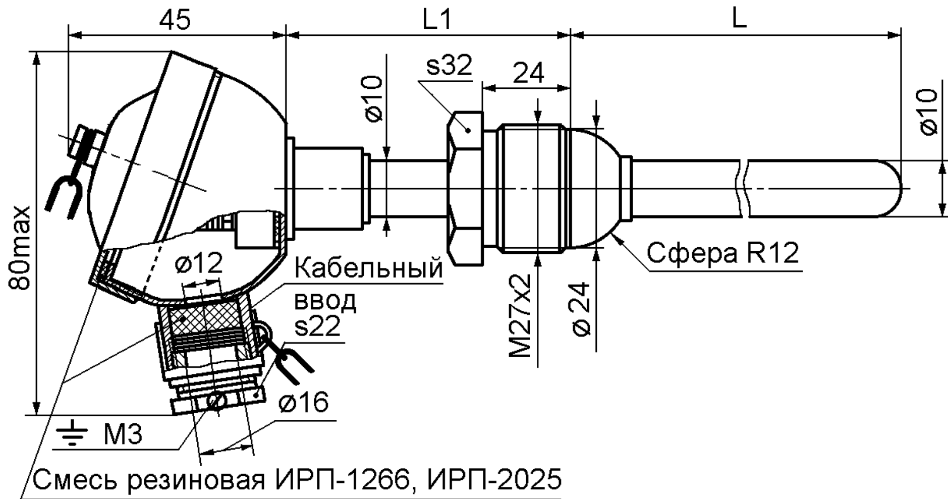
Рисунок Г.4 – Штуцер подвижный
