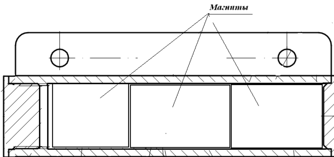
Рисунок 1. Конструкция Извещателей модели 01, 02.
