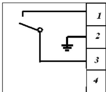
в) Схема внутренних соединений Извещателей модели 01
