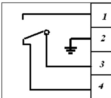
г) Схема внутренних соединений Извещателей модели 02
