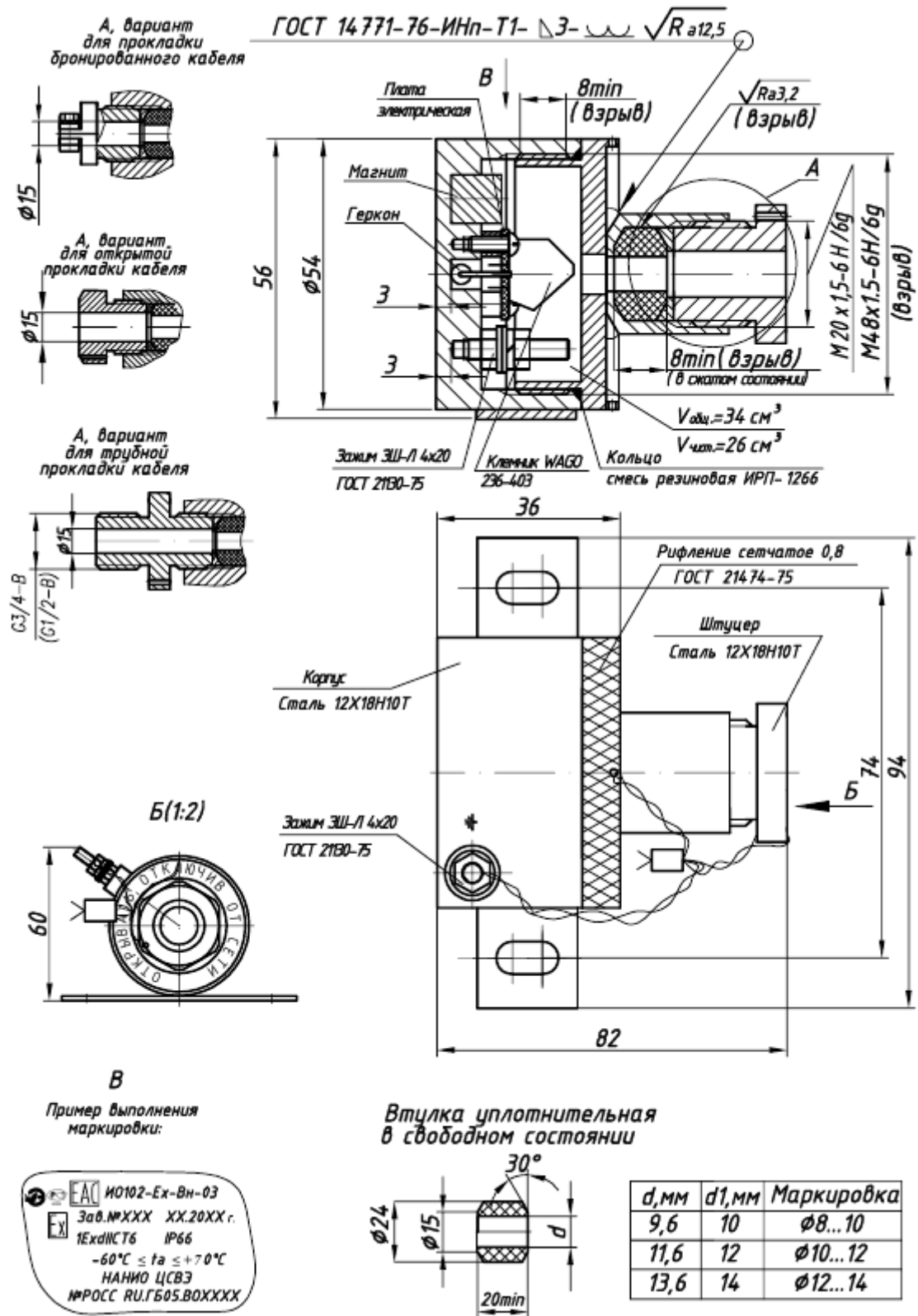
Рисунок А2 Габаритный чертёж Извещателей моделей 03.
