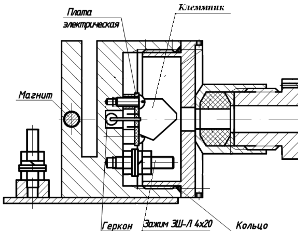
Рисунок 3 . Конструкция Извещателей модели 04
