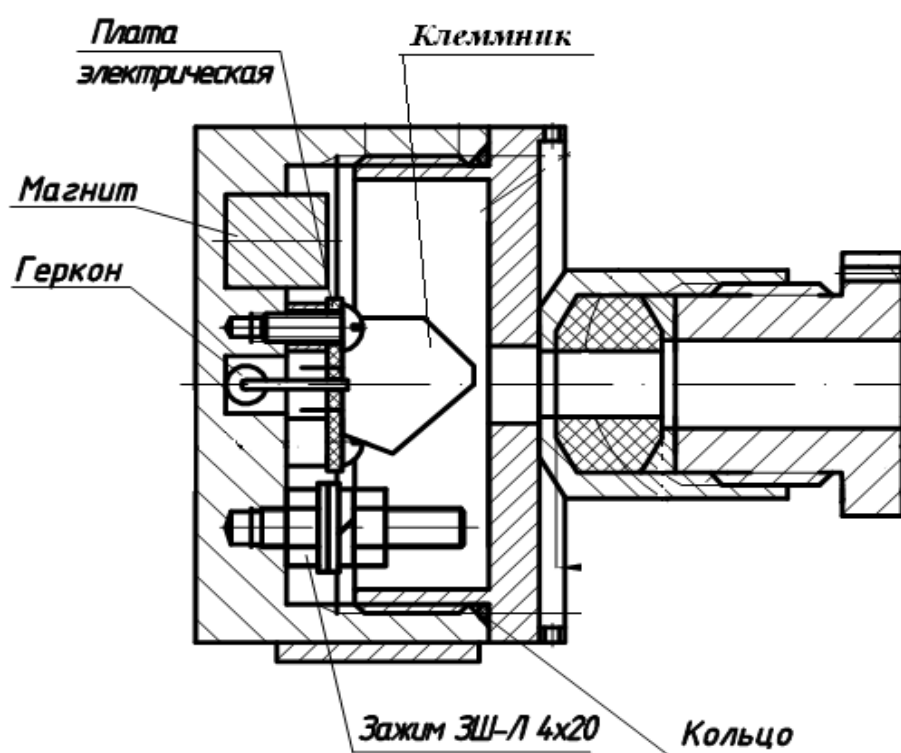
Рисунок 2 . Конструкция Извещателей модели 03
