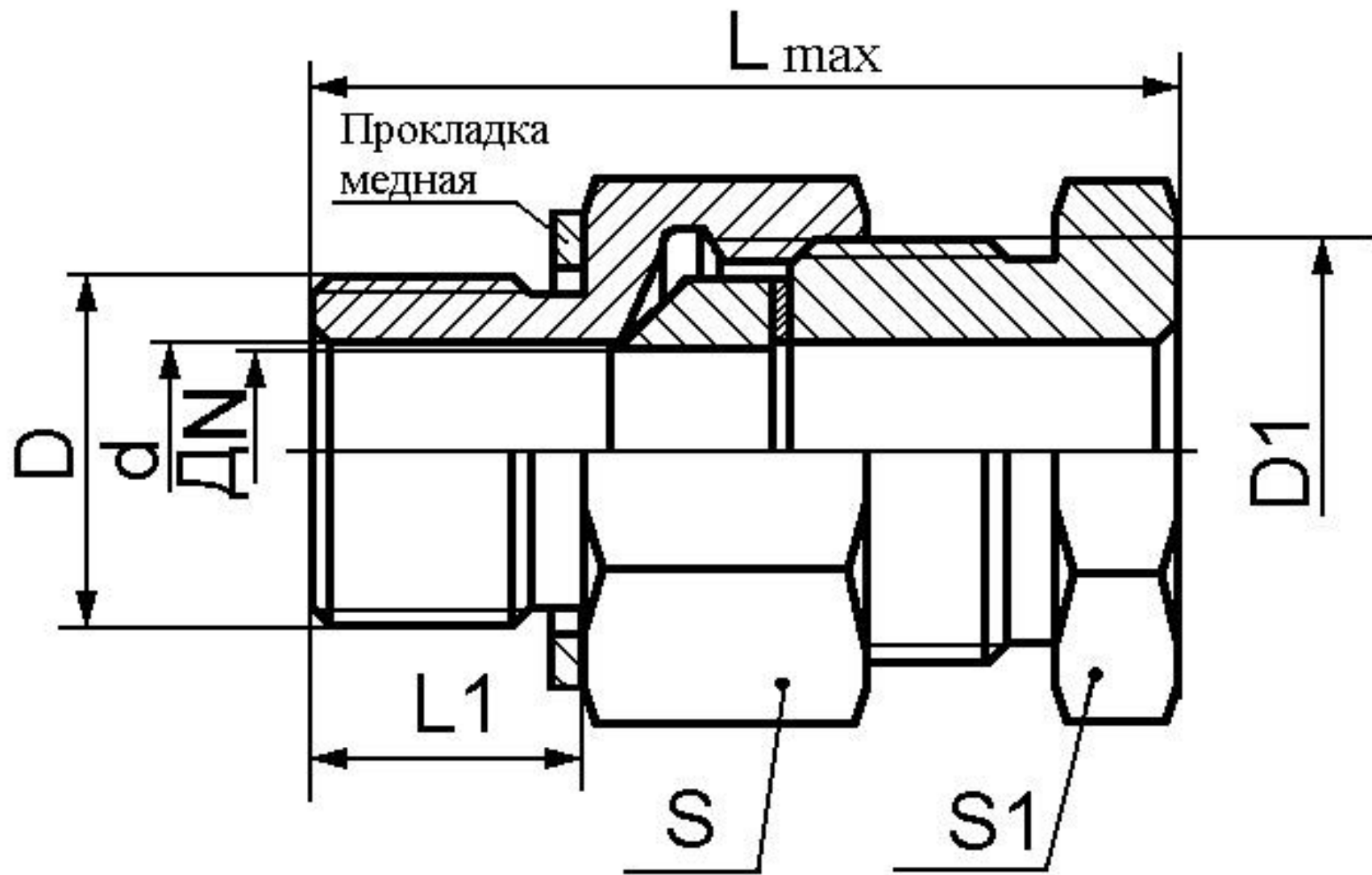
Рисунок 2 – Штуцер передвижной. Температурный диапазон от минус 60 до плюс 500 °С
