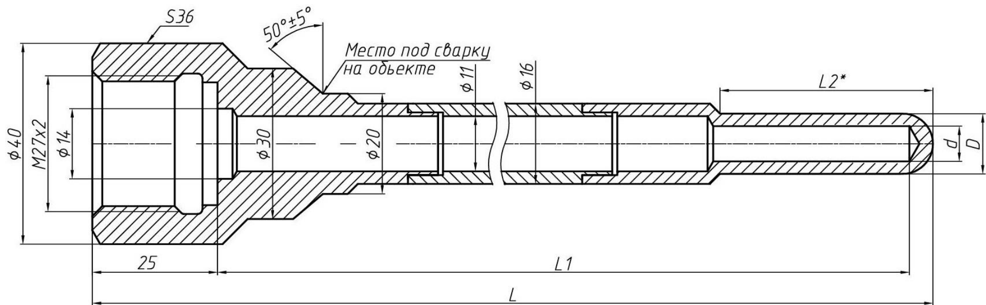
Рисунок 3 – Гильза ГЗВ-8040 (ЮВМА.408721.162)
