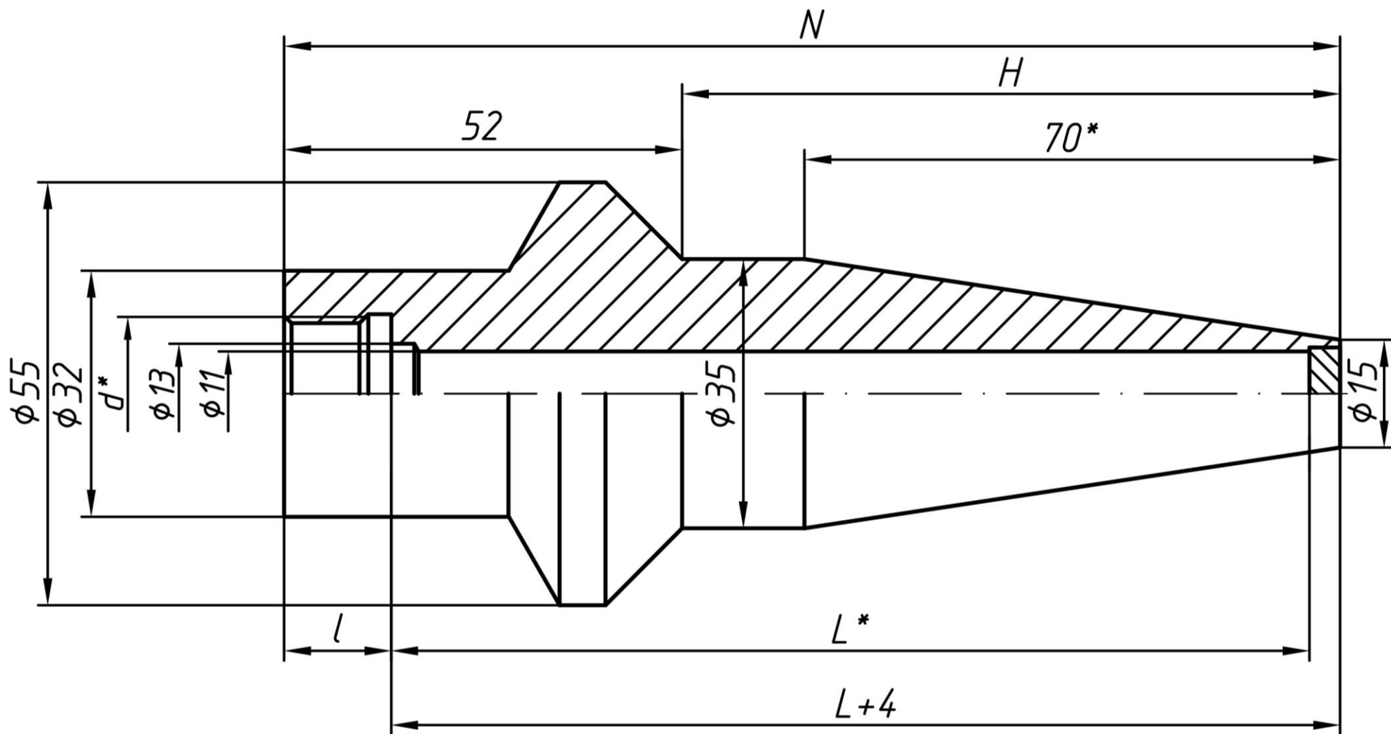
Рисунок 1 – Гильза ГЗВ - 1
