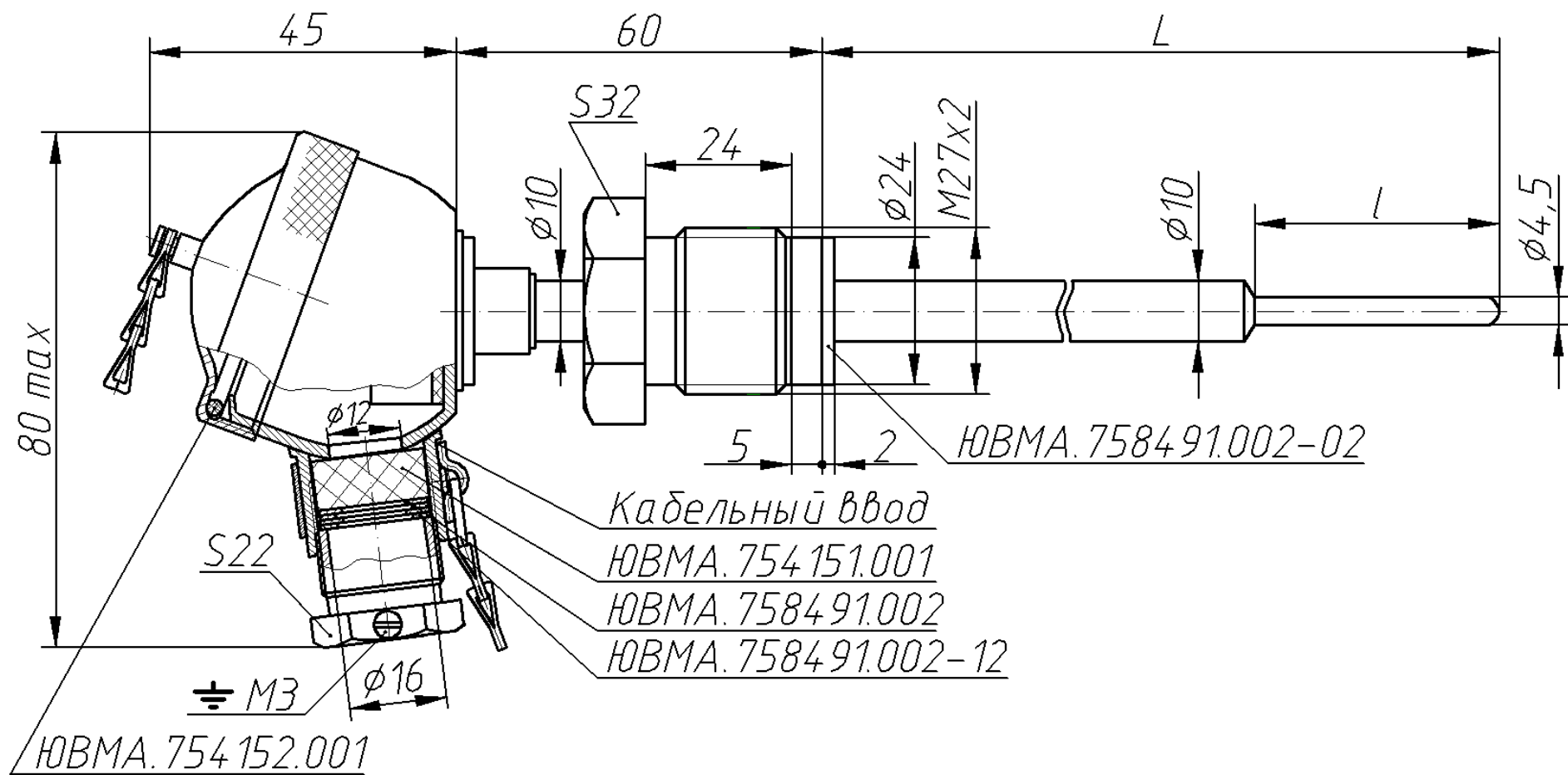
Габаритный чертеж термометра ТСП/1-8041
