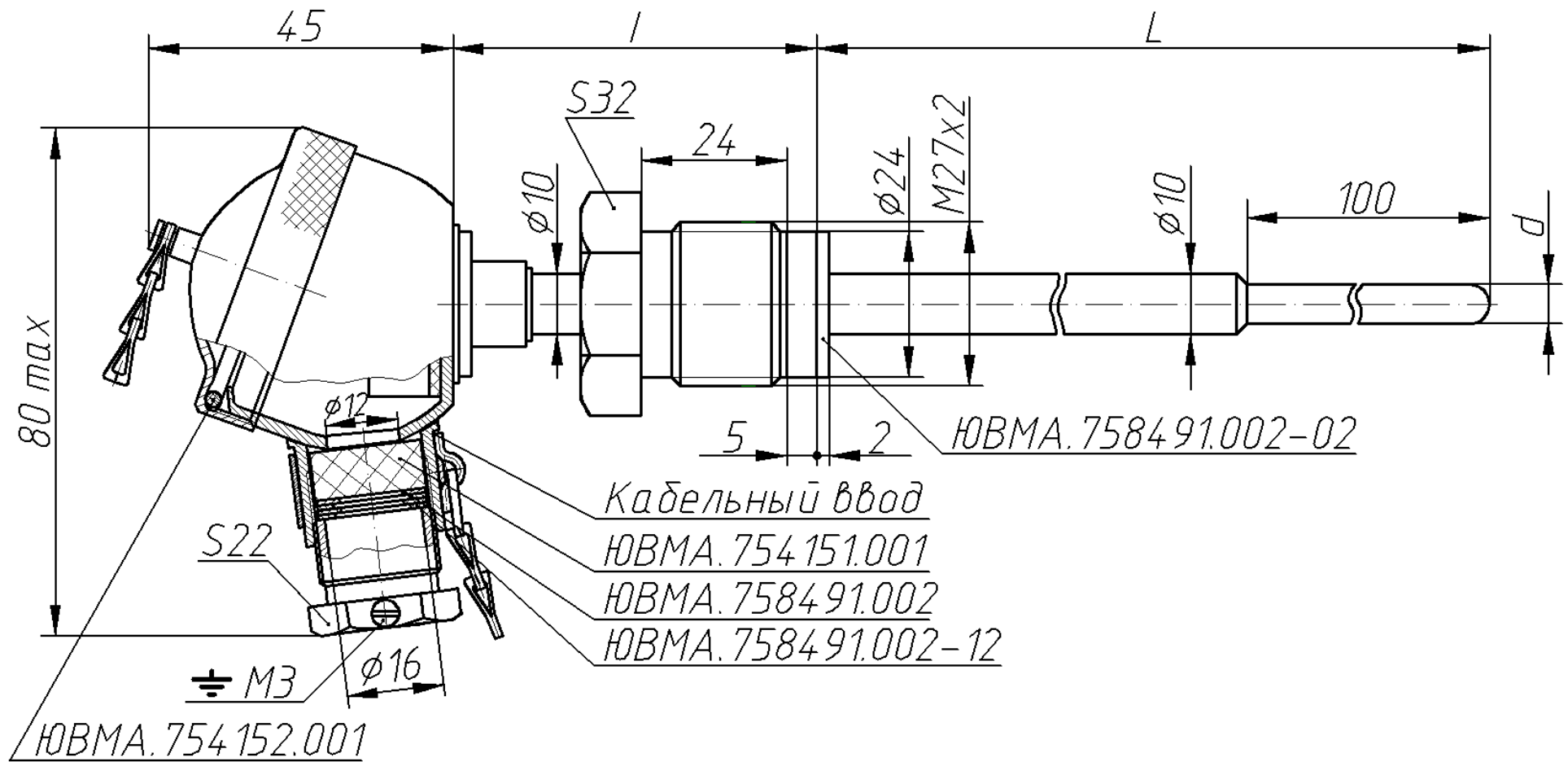
Рисунок В.6 – Штуцер подвижный
