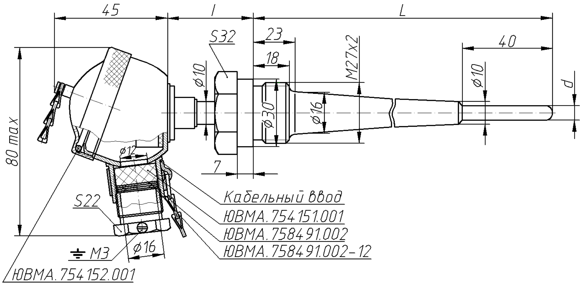
Рисунок В.4 – Штуцер неподвижный
