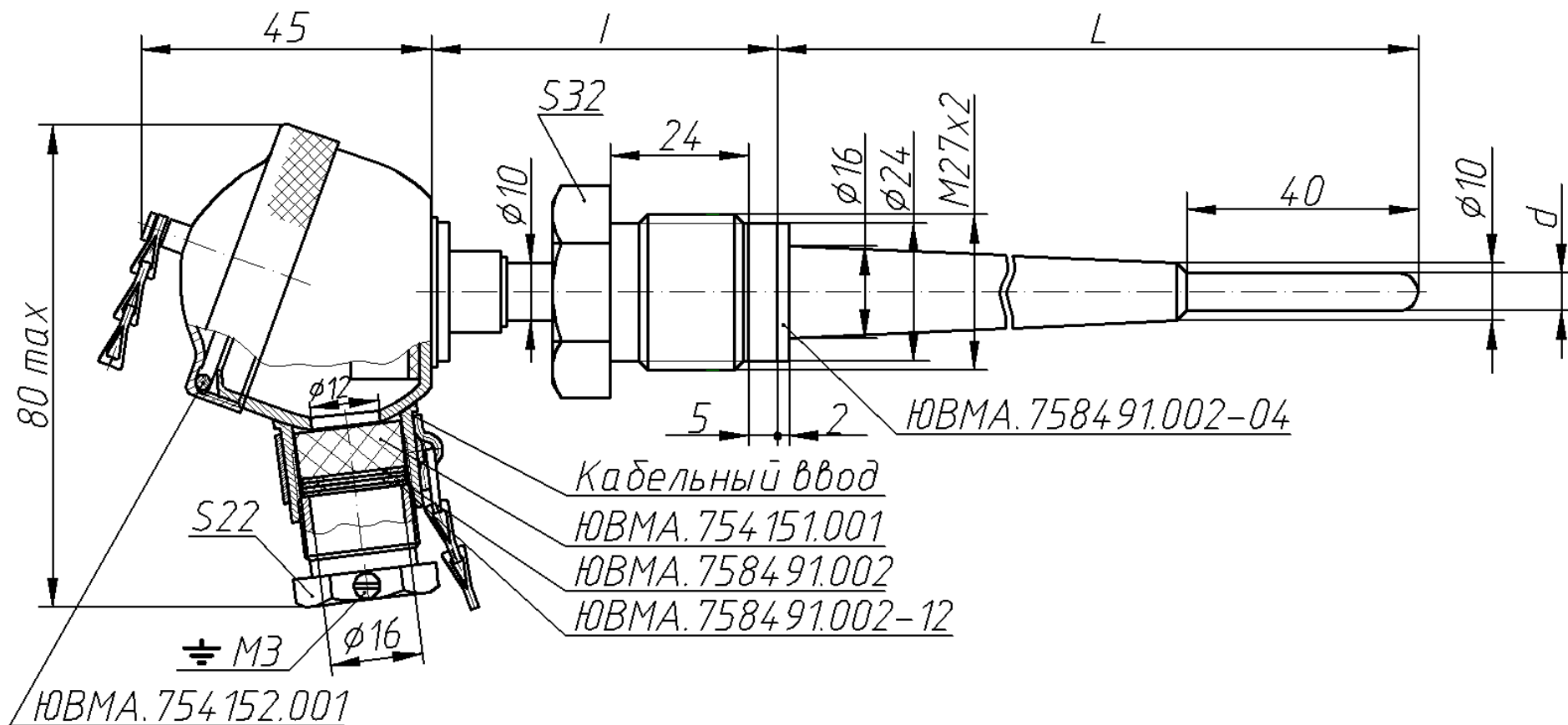
Рисунок В.3 – Штуцер подвижный
