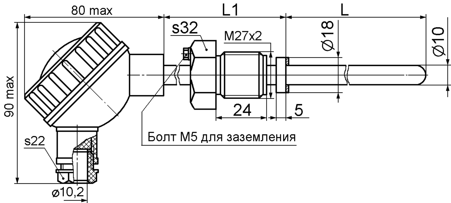
Рисунок В.1 – Штуцер подвижный
