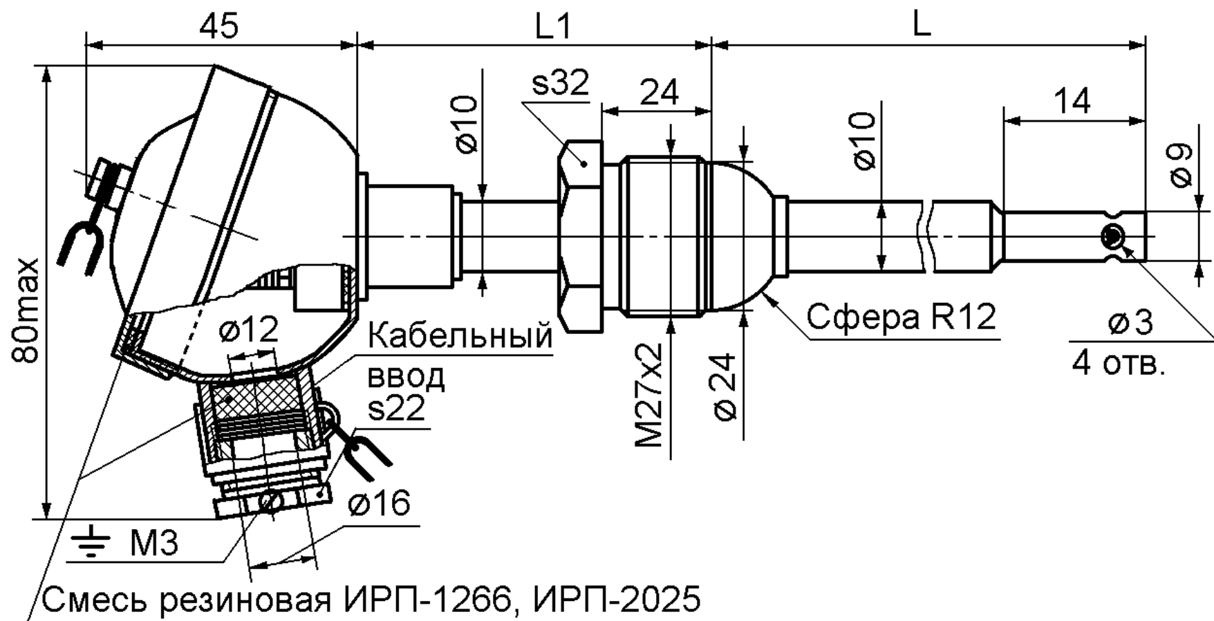
Рисунок Г.5 – Штуцер подвижный
